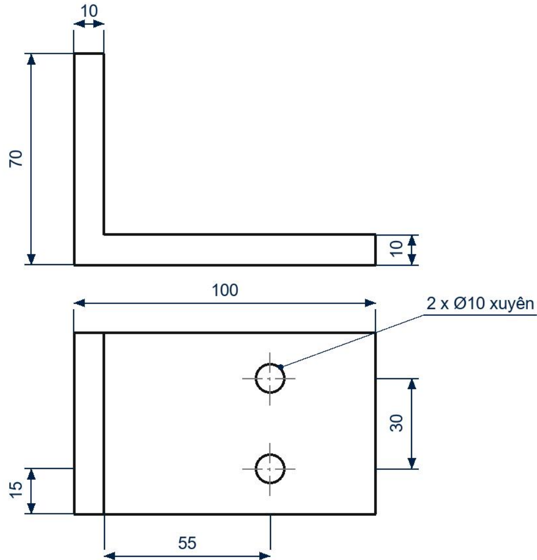
HÌNH CHIẾU ĐỨNG
