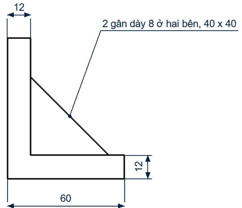
HÌNH CHIẾU CẠNH (TRÁI)
