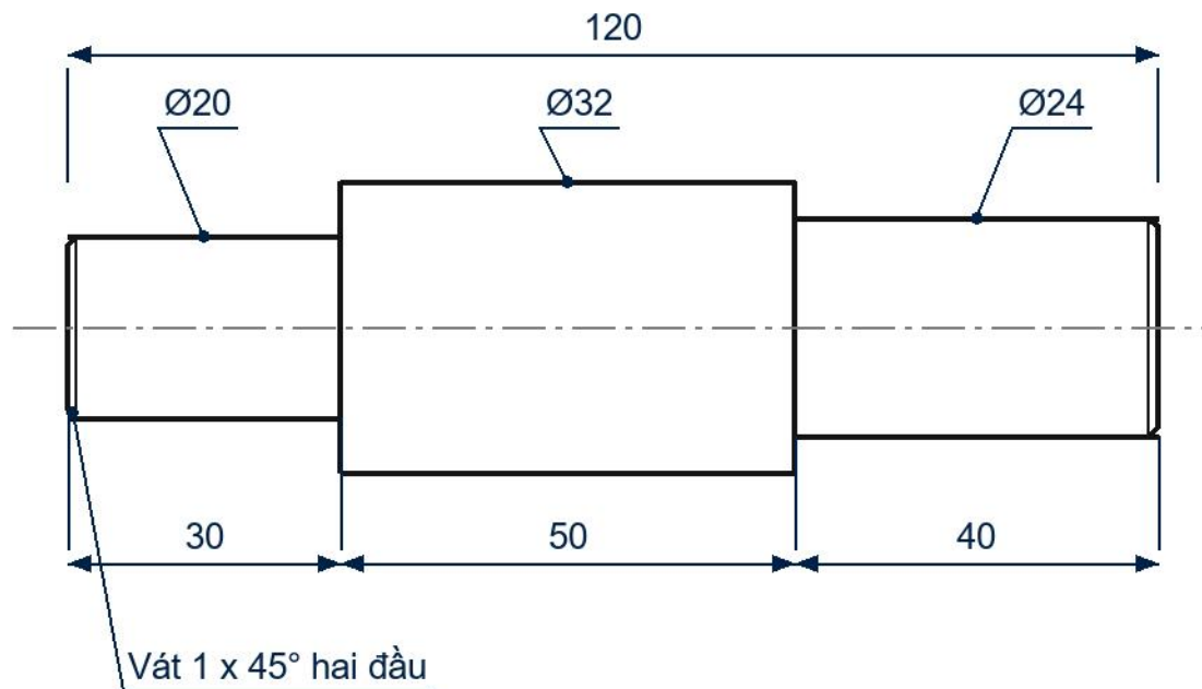
HÌNH CHIẾU ĐỨNG
